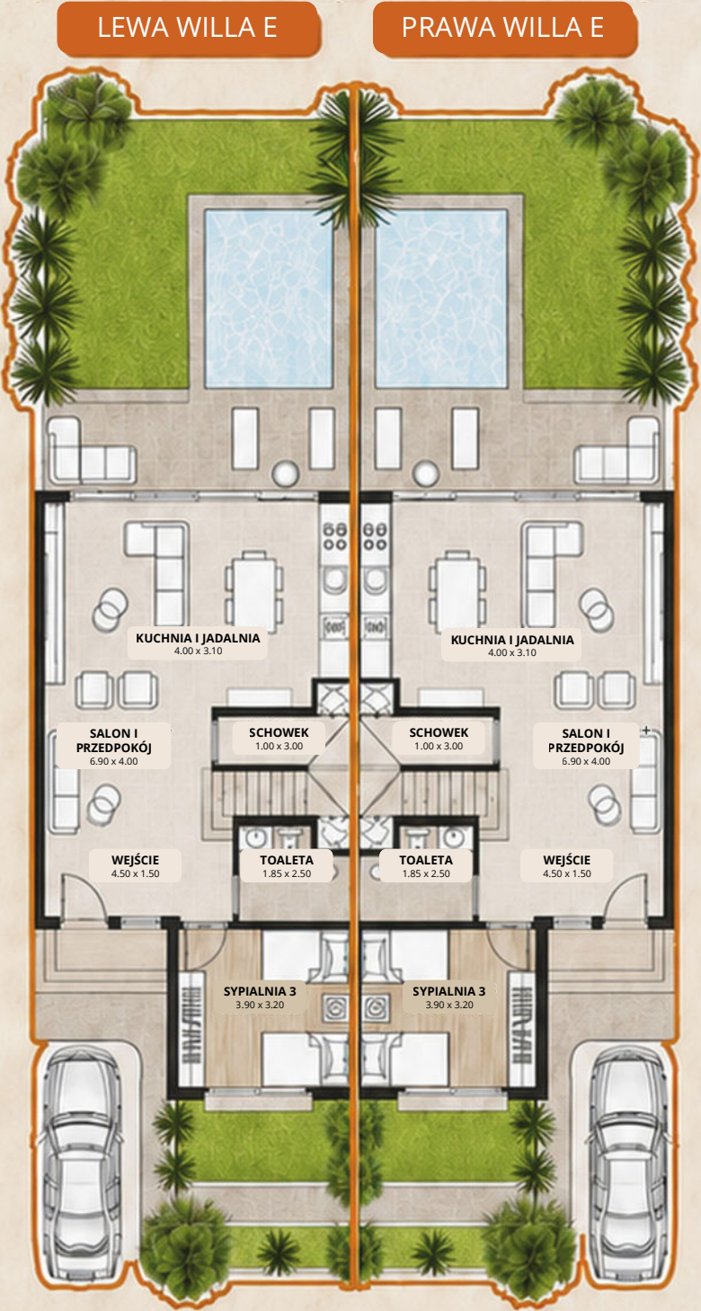
RZUT PARTERU
